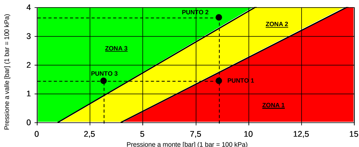
DIAGRAMMA DI CAVITAZIONE *
