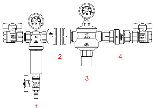
Figura 1: Impianto autonomo unifamiliare: Applicazione dell'anticalcare sull'alimentazione generale.
