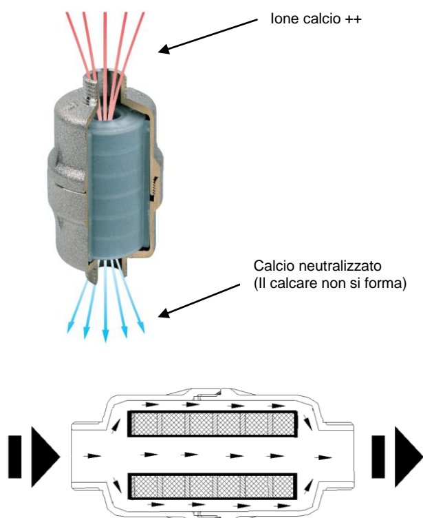
Schema passaggio del fluido attraverso l'Anticalcare magnetico
